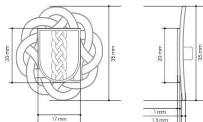
TEHNISKAIS ZĪMĒJUMS
